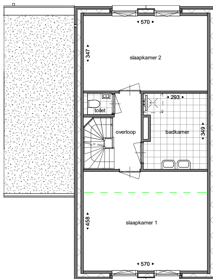
eerste verdieping
