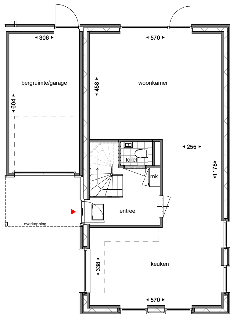
begane grond
