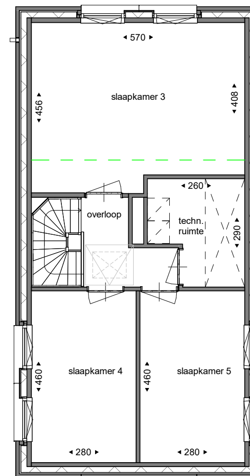
tweede verdieping
